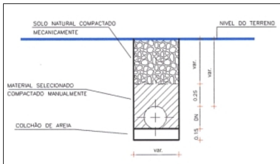
Figura 1 - Esquema de valas e assentamento de tubos.
